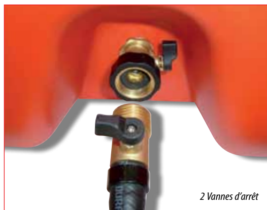
Pompe intégrée
